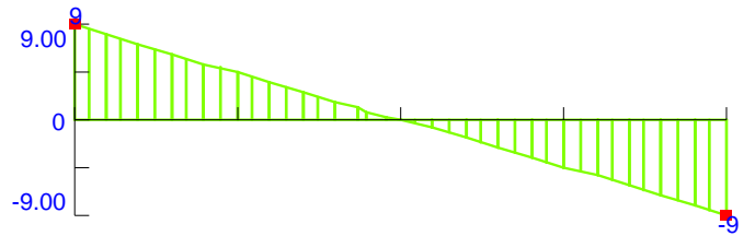
Shear Diagram (Y) (kip)
